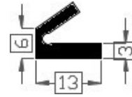
Art.2017806 TPE 60° shore zwart Gewicht ca. 90 gr/mt
