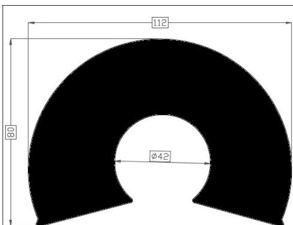
Art.2015262 TPE 60° shore zwart Gewicht ca. 5408 gr/mt
