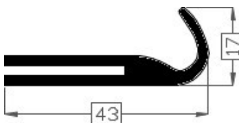
Art.20181133 TPE 60° shore zwart Gewicht ca. 220 gr/mt
