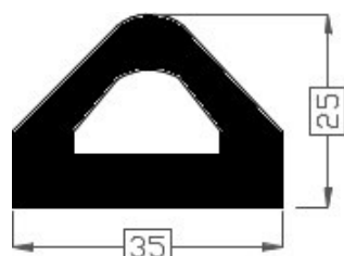
Art.2016379 TPE 60° shore zwart Gewicht ca. 560 gr/mt
