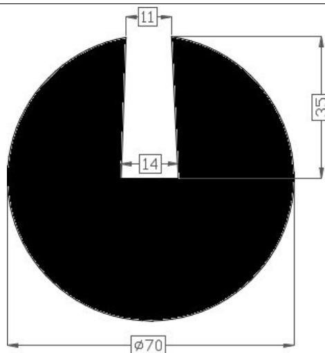
Art.20181153 TPE 60° shore zwart Gewicht ca. 3215 gr/mt
