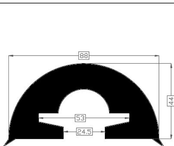
Art.2014060 TPE 60° shore zwart Gewicht ca. 2500 gr/mt
