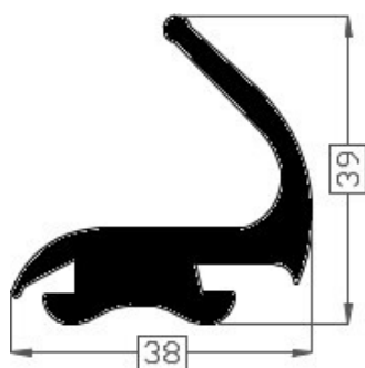
Art.2017852 TPE 60° shore zwart Gewicht ca. 380 gr/mt
