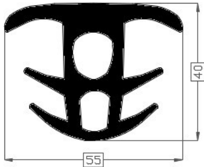
Art.20181269 TPE 60° shore zwart Gewicht ca..875 gr/mt
