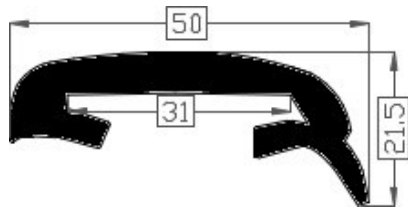
Art.20181201 TPE 60° shore zwart Gewicht ca. 385 gr/mt
