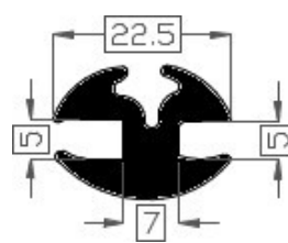
Art.2016507 TPE 60° shore zwart Gewicht ca. 217 gr/mt
