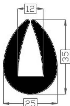
Art.2017891 TPE 60° shore zwart Gewicht ca. 495 gr/mtr
