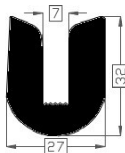
Art.2017755 TPE 60° shore zwart Gewicht ca. 640 gr/mtr
