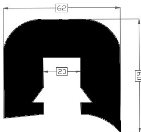
Art.2015097 TPE 60° shore zwart Gewicht ca. 2342 gr/mt
