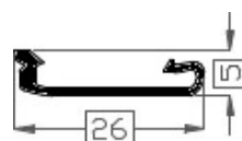
Art.20181282 TPE 60° shore zwart Gewicht ca. 45 gr/mt
