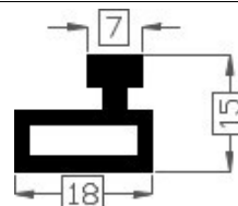
Art.2016338 TPE 60° shore zwart Gewicht ca. 122 gr/mt
