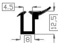
Art.2014048 TPE 60° shore zwart Gewicht ca. 84 gr/mt
