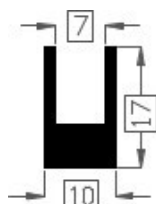
Art.20181121 TPE 60° shore zwart Gewicht ca. 150 gr/mt
