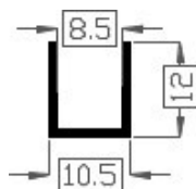
Art.20181223 TPE 60° shore zwart Gewicht ca. 35 gr/mt
