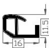
Art.20181410 TPE 60° shore zwart Gewicht ca. 80 gr/mt
