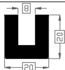
Art.20181204 TPE 60° shore zwart Gewicht ca. 276 gr/mt
