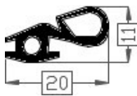
Art.2017977 TPE 60° shore zwart Gewicht ca. 95 gr/mt
