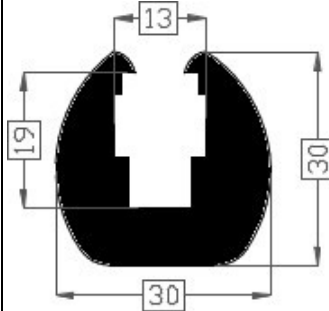
Art.2014030 TPE 60° shore zwart Gewicht ca. 505 gr/mtr
