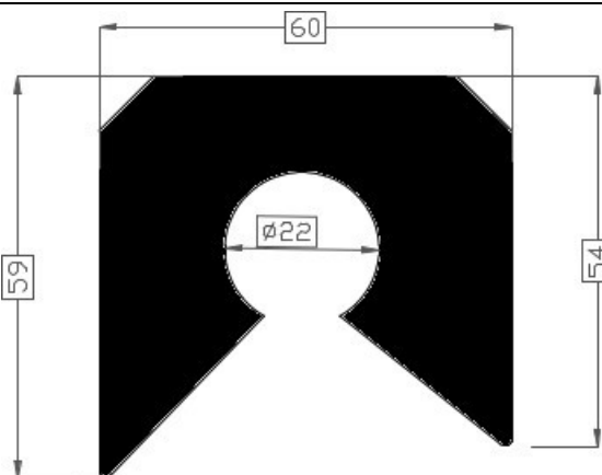
Art.2015137 TPE 60° shore zwart Gewicht ca. 2350 gr/mt
