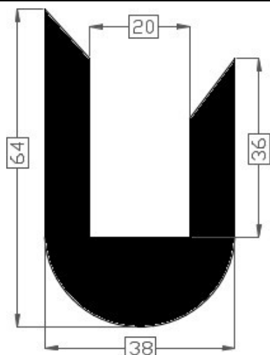
Art.20181087 TPE 60° shore zwart Gewicht ca. 1310 gr/mt
