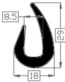
Art.20181307/70 TPE 70° shore zwart Gewicht ca. 205 gr/mtr
