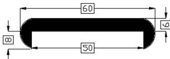
Art.20181142 TPE 60° shore zwart Gewicht ca.500 gr/mt
