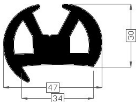
Art.2014072 In combinatie met art: 2015120 TPE 60° shore zwart Gewicht ca. 790 gr/mt
