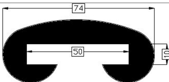
Art.2014056 TPE 60° shore zwart Gewicht ca. 1160 gr/mt
