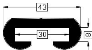
Art.2017796 TPE 60° shore zwart Gewicht ca. 475 gr/mt
