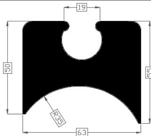
Art.2016380 TPE 60° shore zwart Gewicht ca. 2027 gr/mt
