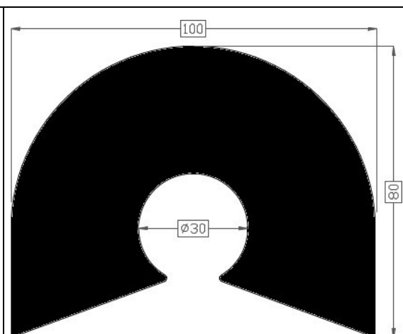
Art.2016580 TPE 60° shore zwart Gewicht ca. 5530 gr/mt
