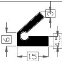
Art.2017905/20 TPE 20° shore zwart Gewicht ca. gr/mt
