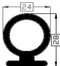
Art.2014624 TPE 60° shore zwart Gewicht ca. 281 gr/mt
