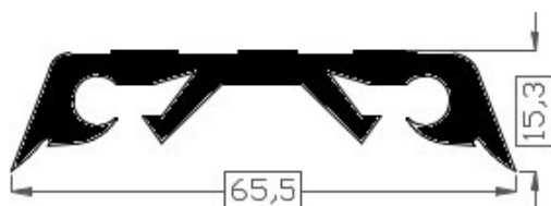
Art.2015146/70 TPE 70° shore zwart Gewicht ca. 495 gr/mt
