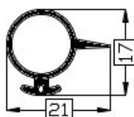
Art.2014627 TPE 60° shore zwart Gewicht ca. 75 gr/mt
