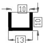
Art.2014662 TPE 60° shore zwart Gewicht ca. 49 gr/mt
