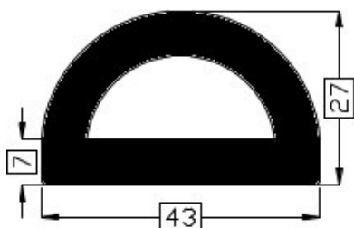
Art.2015104/70 TPE 70° shore zwart Gewicht ca. 680 gr/mt
