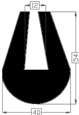
Art.2017723/70 TPE 70° shore zwart Gewicht ca. 1365 gr/mtr
