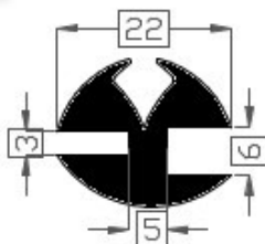
Art.2015132 TPE 60° shore zwart Gewicht ca. 225 gr/mt
