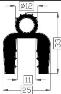
Art.2016341/40 TPE 40° shore zwart Gewicht ca. 400 gr/mt
