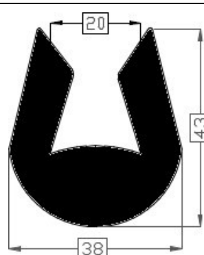
Art.2015189 TPE 60° shore zwart Gewicht ca. 954 gr/mtr
