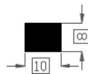
Art.2016510 TPE 60° shore zwart Gewicht ca. 75 gr/mt
