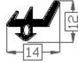
Art.2016469 TPE 60° shore zwart Gewicht ca 45 gr/mt
