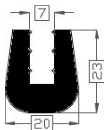
Art.2015219 TPE 60° shore zwart Gewicht ca. 288 gr/mtr
