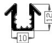
Art.2015197 TPE 60° shore zwart Gewicht ca. 76 gr/mt
