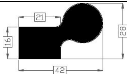
Art. 20181296 TPE 60° shore zwart Gewicht ca..780 gr/mt
