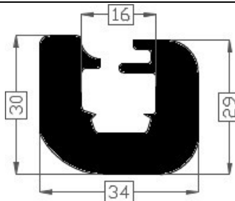
Art.2015208 TPE 60° shore zwart Gewicht ca. 706 gr/mtr
