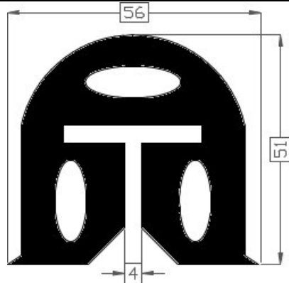
Art.2017751 TPE 60° shore zwart Gewicht ca. 1428 gr/mt
