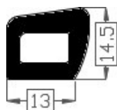
Art.2016386 TPE 60° shore zwart Gewicht ca. 125 gr/mt
