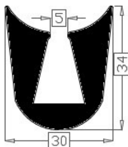
Art.20181162 TPE 60° shore zwart Gewicht ca. 625 gr/mtr
