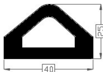
Art.2014036 TPE 60° shore zwart Gewicht ca. 540 gr/mt
