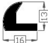
Art.2016536 TPE 60° shore zwart Gewicht ca 110 gr/mt
