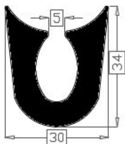
Art.2015123 TPE 60° shore zwart Gewicht ca. 560 gr/mtr
