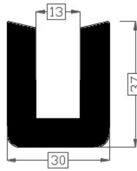
Art.2015087 TPE 60° shore zwart Gewicht ca. 763 gr/mt
