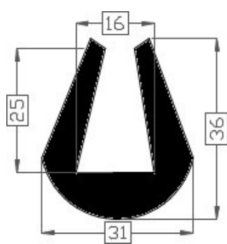
Art.2016391 TPE 60° shore zwart Gewicht ca. 570 gr/mtr
