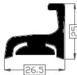
Art.20181132 TPE 60° shore zwart Gewicht ca. 280 gr/mt
