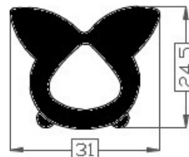
Art.2015320 TPE 60° shore zwart Gewicht ca. 409 gr/mt
