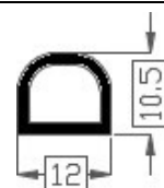
Art.20181062/20 TPE 20° shore zwart Gewicht ca. 75 gr/mt
