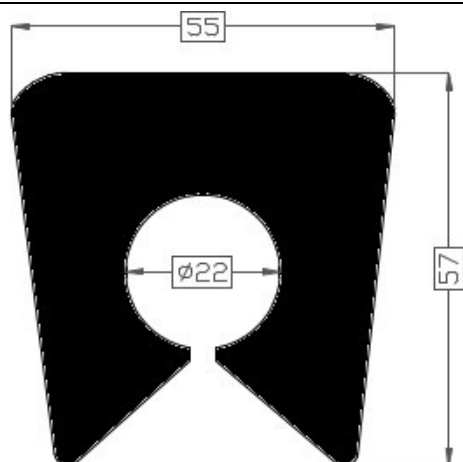
Art.2014628 TPE 60° shore zwart Gewicht ca. 2210 gr/mt
