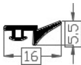
Art.20181321 TPE 60° shore zwart Gewicht ca. 35 gr/mt
