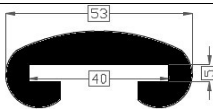
Art.2017803 TPE 60° shore zwart Gewicht ca. 665 gr/mt
