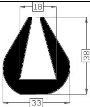
Art.2015173 TPE 60° shore zwart Gewicht ca. 610 gr/mtr
