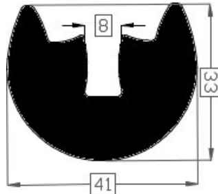
Art.2015277/70 TPE 70° shore zwart Gewicht ca. 810 gr/mt
