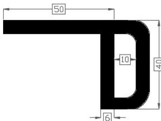
Art.20181273 TPE 60° shore zwart Gewicht ca. 925 gr/mt
