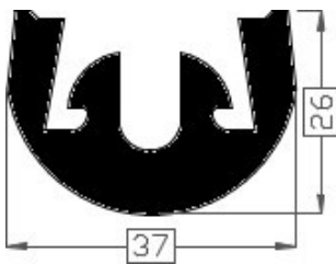
Art.2017869 TPE 60° shore zwart Gewicht ca. 525 gr/mtr
