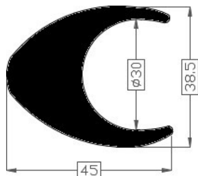
Art.2017774 TPE 60° shore zwart Gewicht ca. 820 gr/mt
