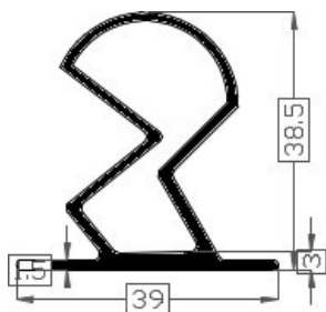
Art.20181024 TPE 60° shore zwart Gewicht ca. 330 gr/mt
