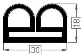
Art.20181324/20 TPE 20° shore zwart Gewicht ca. 325 gr/mt
