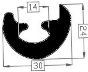
Art.2015213 TPE 60° shore zwart Gewicht ca. 357 gr/mtr
