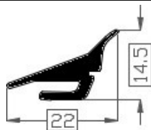
Art.20181115 TPE 60° shore zwart Gewicht ca. 95 gr/mt
