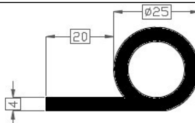
Art.2015249 TPE 60° shore zwart Gewicht ca. 375 gr/mt
