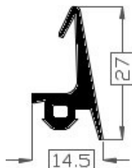
Art.2016433 TPE 60° shore zwart Gewicht ca. 105 gr/mt
