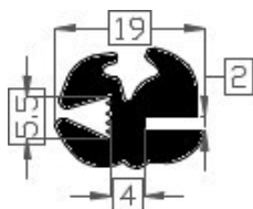
Art.20181095 TPE 60° shore zwart Gewicht ca. 180 gr/mt
