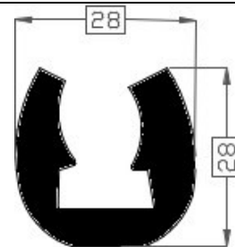
Art.2015226 TPE 60° shore zwart Gewicht ca. 1040 gr/mt
