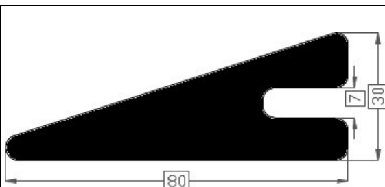
Art.20181102 TPE 60° shore zwart Gewicht ca. 1355 gr/mt
