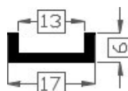
Art.20181048 TPE 60° shore zwart Gewicht ca.60 gr/mt
