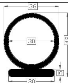
Art.20181169 TPE 60° shore zwart Gewicht ca. 475 gr/mt
