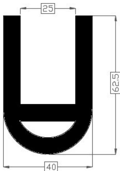
Art.20181087 TPE 60° shore zwart Gewicht ca. 1310 gr/mt
