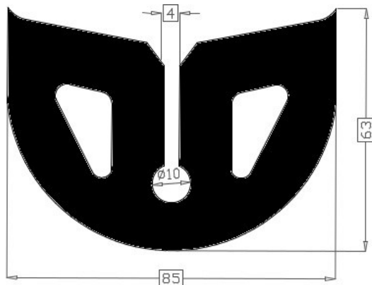
Art.2015109/70 TPE 70° shore zwart Gewicht ca. 3322 gr/mt
