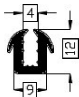
Art.2014663 TPE 60° shore zwart Gewicht ca. 74 gr/mt
