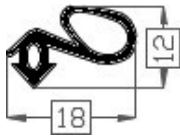
Art.2016344 TPE 60° shore zwart Gewicht ca. 82 gr/mt
