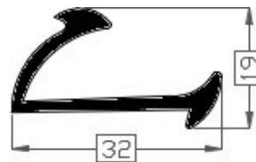
Art.2016551 TPE 60° shore zwart Gewicht ca 140 gr/mt
