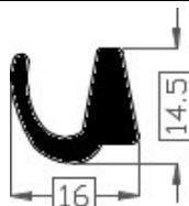
Art.20181364 TPE 60° shore zwart Gewicht ca.110 gr/mt
