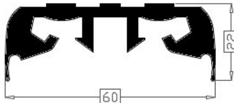
Art.2016395 TPE 60° shore zwart Gewicht ca. 525 gr/mt
