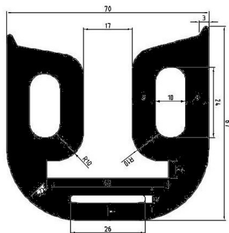
Art2014635 TPE 60° shore zwart Gewicht ca. 2874 gr/mt
