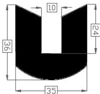
Art.2014644 (LM) TPE 60° shore zwart Gewicht ca. 900 gr/mt
