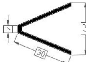
Art.2017598 TPE 60° shore zwart Gewicht ca. 132 gr/mt
