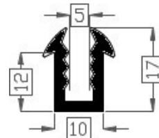
Art.2014049 TPE 60° shore zwart Gewicht ca. 88 gr/mt
