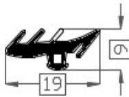
Art.20181332 TPE 60° shore zwart Gewicht ca. 75 gr/mt
