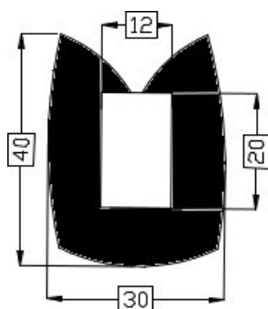
Art.2014023 TPE 60° shore zwart Gewicht ca. 825 gr/mt
