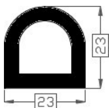
Art.20181225 TPE 60° shore zwart Gewicht ca. 300 gr/mt
