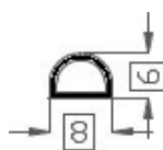
Art.20181060 TPE 60° shore zwart Gewicht ca. 35 gr/mt
