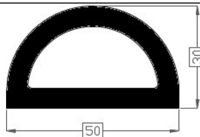
Art.20181097/70 TPE 70° shore zwart Gewicht ca. 850 gr/mt
