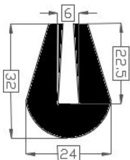
Art.2014042 TPE 60° shore zwart Gewicht ca. 516 gr/mtr
