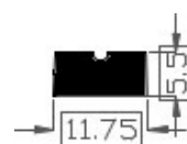
Art.20181377 TPE 60° shore zwart Gewicht ca. 56 gr/mt
