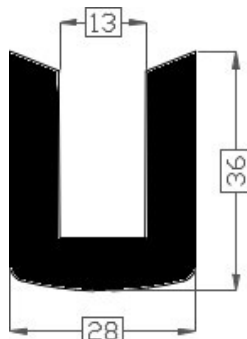
Art.2016400/90 TPE 90° shore zwart Gewicht ca. 645 gr/mt
