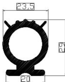
Art.2015126 TPE 60° shore zwart Gewicht ca. 291gr/mt
