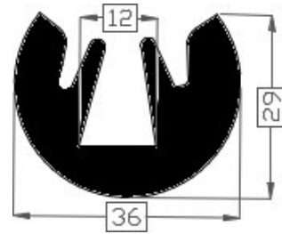
Art.2015176 TPE 60° shore zwart Gewicht ca. gr/mt
