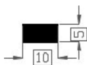
Art.2017732 TPE 60° shore zwart Gewicht ca. 48 gr/mt
