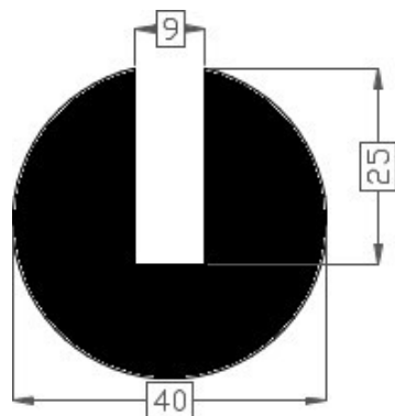
Art.2016498 TPE 60° shore zwart Gewicht ca. 905 gr/mt
