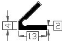
Art.2017814 TPE 60° shore zwart Gewicht ca. 55 gr/mt
