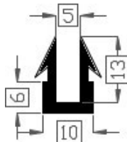
Art.2015089 TPE 60° shore zwart Gewicht ca. 85 gr/mt
