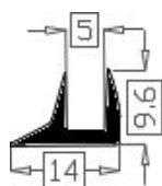
Art.2014614 TPE 60° shore zwart Gewicht ca. 110 gr/mt
