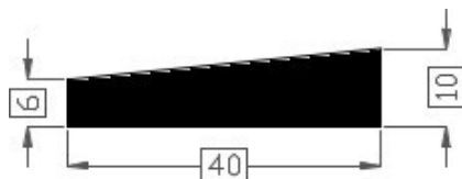
Art.20181192/40 TPE 40° shore zwart Gewicht ca. 325 gr/mt
