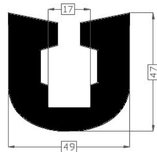
Art.2014609 (o.a Saga) TPE 60° shore zwart Gewicht ca. 1555 gr/mtr
