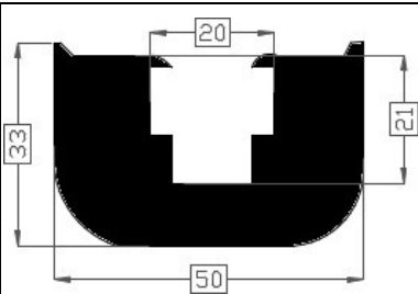
Art.2014052 TPE 60° shore zwart Gewicht ca. 1100 gr/mtr
