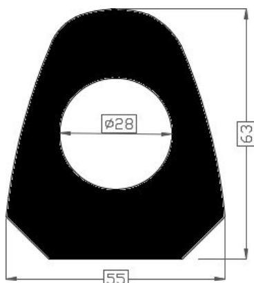
Art.2016432/40 TPE 40° shore zwart Gewicht ca. 1760 gr/mtr
