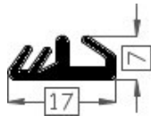
Art.20181066 TPE 60° shore zwart Gewicht ca. 60 gr/mt
