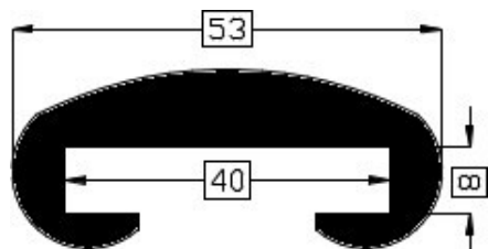
Art.2014672/70 TPE 70° shore zwart Gewicht ca. 695 gr/mt
