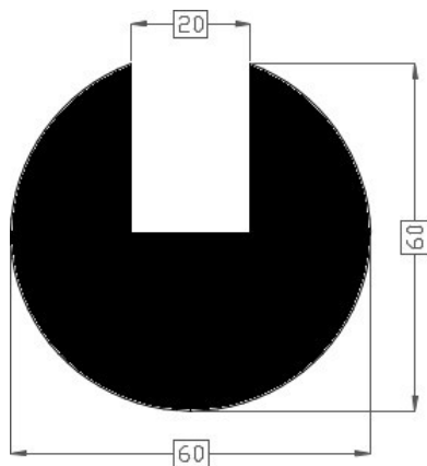
Art.2016366/70 TPE 70° shore zwart Gewicht ca. 2100 gr/mt
