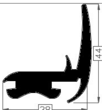
Art.2017853 TPE 60° shore zwart Gewicht ca. 525 gr/mt
