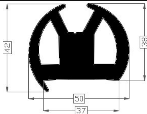
Art.2015119 In combinatie met art: 2015120 TPE 60° shore zwart Gewicht ca. 790 gr/mt
