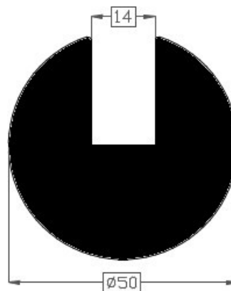
Art.2017897 TPE 60° shore zwart Gewicht ca. 1650 gr/mt
