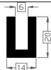
Art.20181391 TPE 60° shore zwart Gewicht ca. 185 gr/mt
