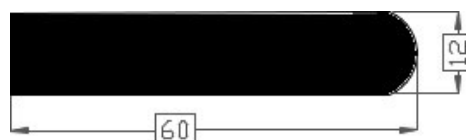
Art.2016456/50 TPE 50° shore zwart Gewicht ca. 700 gr/mt
