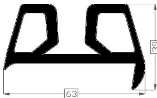
Art.2017857 TPE 60° shore zwart Gewicht ca. 850 gr/mt
