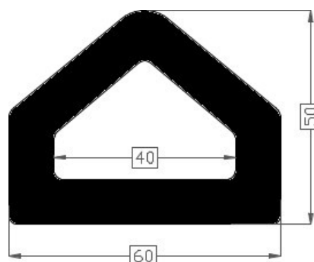
Art.2014017 TPE 60° shore zwart Gewicht ca. 1550 gr/mt
