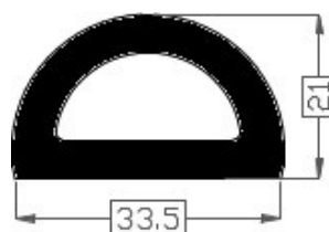
Art.2017771/70 TPE 70° shore zwart Gewicht ca. 375 gr/mt
