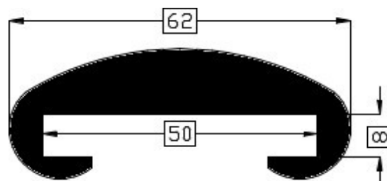
Art.2014041 TPE 60° shore zwart Gewicht ca. 717 gr/mt
