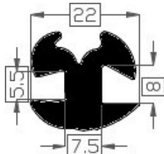
Art.2015212 TPE 60° shore zwart Gewicht ca. 237 gr/mt
