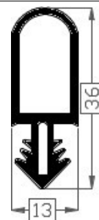
Art.20181202 TPE 60° shore zwart Gewicht ca. 165 gr/mt
