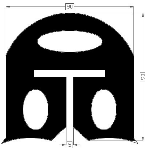
Art.2017935 TPE 60° shore zwart Gewicht ca. 5200 gr/mt
