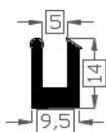
Art.2015122 TPE 60° shore zwart Gewicht ca. 78 gr/mt
