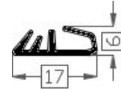
Art.20181112 TPE 60° shore zwart Gewicht ca.40 gr/mt
