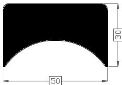
Art.2016506 TPE 60° shore zwart Gewicht ca. 1015 gr/mt
