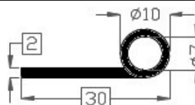
Art.2015264 TPE 60° shore zwart Gewicht ca. 104 gr/mt
