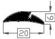
Art.2017855/90 TPE 90° shore zwart Gewicht ca. 70 gr/mt
