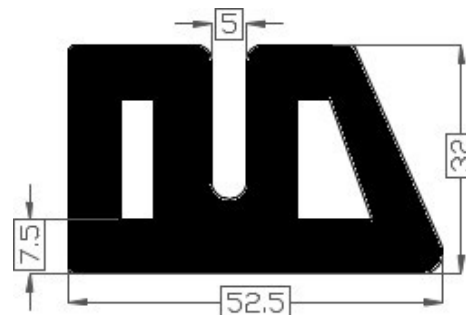
Art.20181354/70 TPE 70° shore zwart Gewicht ca. 1200 gr/mt
